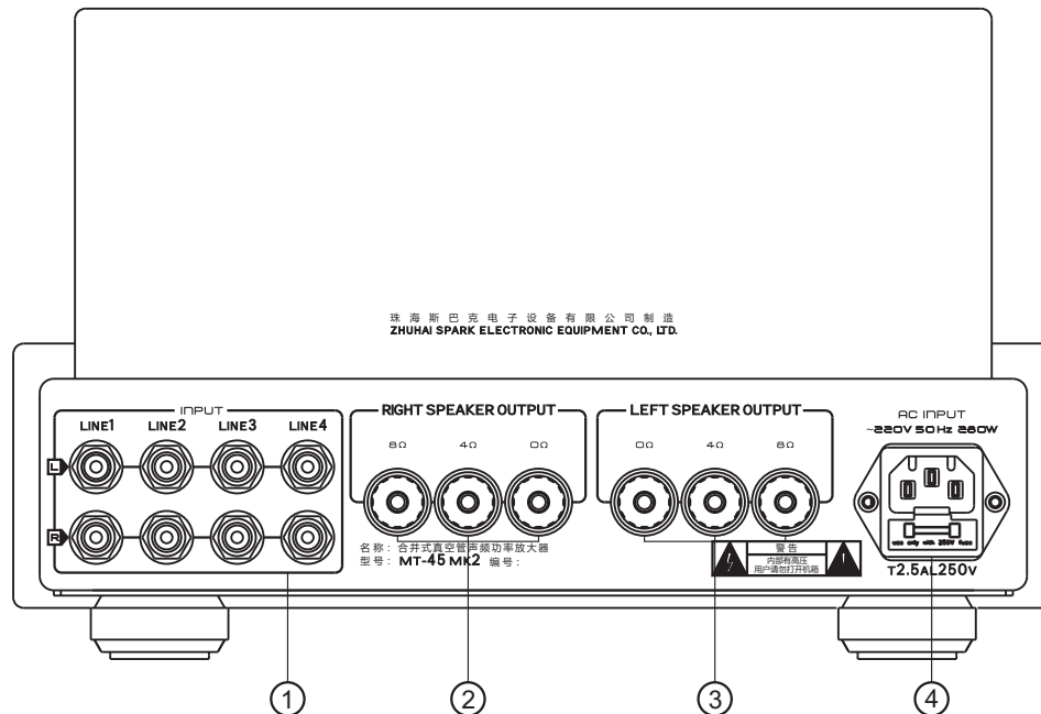
图二：MT-45 MK2后板图
