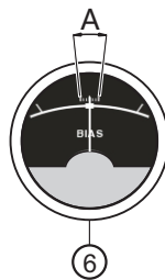
图五： BIAS表工作时指针指示位置图 备注：BIAS表中心刻度A区域 是正常工作区，工作时，会随 市电的波动而变化
