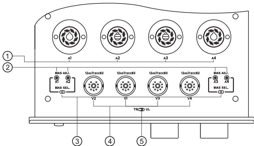
图三：MT-45 MK2顶板图
